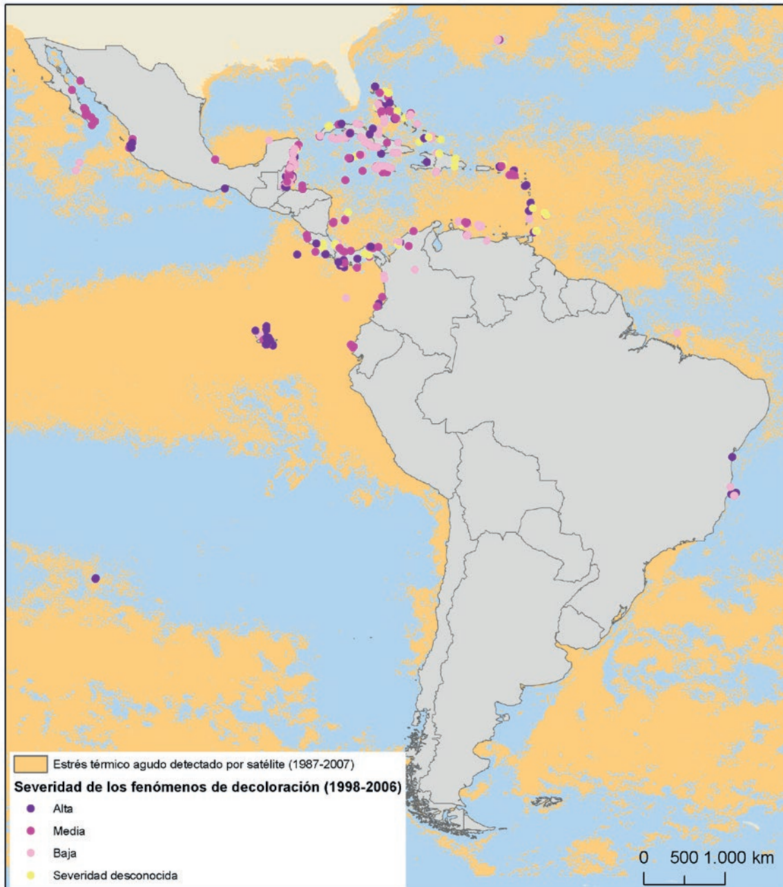
Figura 10.1: Severidad de la decoloración de los arrecifes de coral en América Latina y el Caribe y zonas de alto estrés térmico en los océanos de la región (Reef Base 2014).
