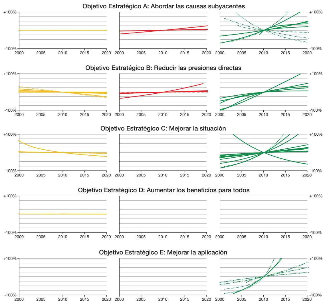
Figura 3: Tendencias de los indicadores normalizados desde el 2000 y proyectados al 2020 para los cinco objetivos diferentes del Plan estratégico para la diversidad biológica 2011-2020 (Tittensor et al. 2014).
