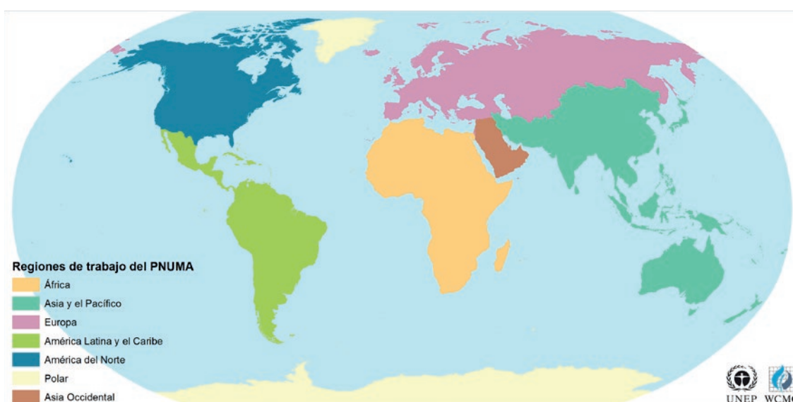
Figura 1: Distribución global de las regiones del UNEP, se muestra la ubicación de la región ALC en verde hierba (mapa elaborado por UNEP-WCMC con datos de Brooks et al. 2016).
