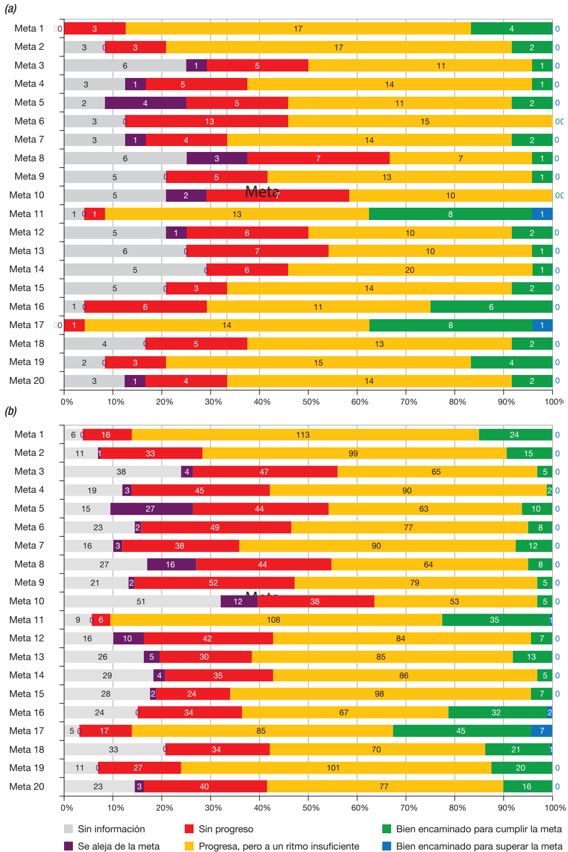
Figura 4: Síntesis del progreso hacia la consecución de las veinte metas de Aichi para la diversidad biológica (a) en todo el mundo y (b) en la región de América Latina y el Caribe. Los números en las columnas indican el número de informes de países dentro de cada categoría, de los 24 informes de países analizados para cada meta.
