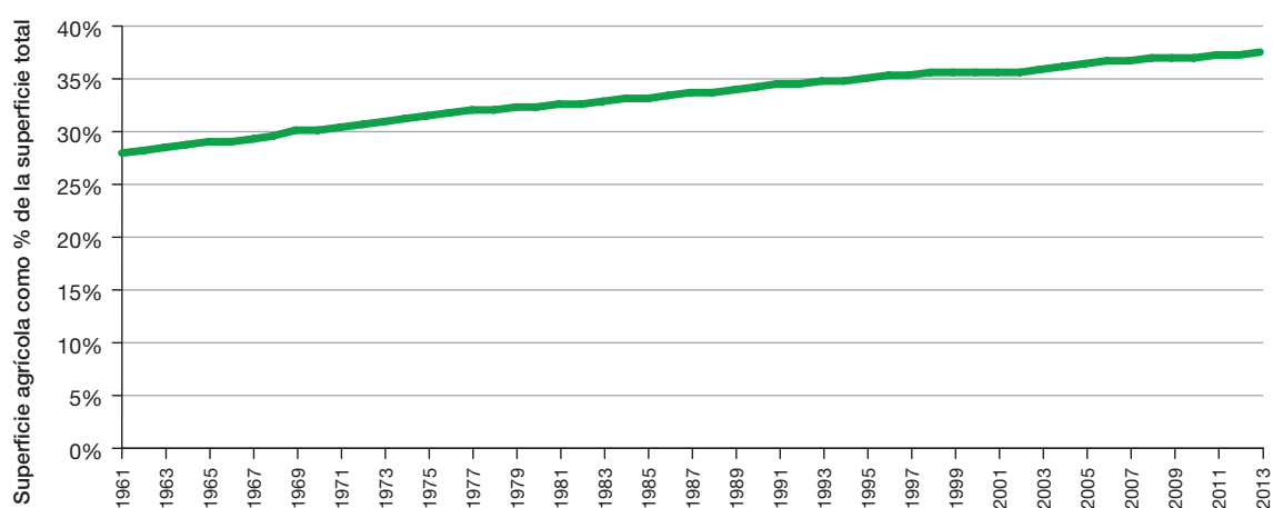
Figura 14.1: Tendencias de la superficie agrícola como % de la superficie total en América Latina y el Caribe entre 1961 y 2010 (fuente: FAO, 2015a).
